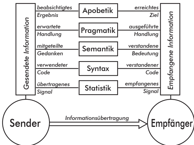
Bild 2: Zum Wesen der Information: Von jeder beliebigen codierten Information gilt, dass sie von jemandem ausgesandt ist (Sender) und an jemanden gerichtet ist (Empfänger). Es sind wesensmäßig fünf verschiedene Ebenen zu unterscheiden. Auf der höchsten Ebene, der Apobetik, geht es um das Informationsziel bzw. -ergebnis. Die darunterliegende Ebene der Pragmatik erfasst die gedachte/bewirkte Handlung. Eine Stufe tiefer geht es um die gedachte/verstandene Bedeutung (Semantik). Die vorletzte Stufe (Syntax) befasst sich mit der sprachlichen Codierung/Decodierung der Gedanken, und die letzte Stufe behandelt das technische Übertragungskonzept und die damit verbundenen statistischen Angaben. Alle fünf Aspekte haben sowohl beim Sender als auch beim Empfänger ihre spezifische Ausprägung. Die einzelnen Ebenen bedingen einander. Das Informationsziel ist nicht erreicht, wenn es auf irgendeiner unteren Ebene zum vorzeitigen Abbruch kommt.
