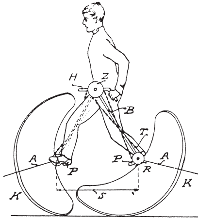
Resim 4: Robert Michael'in viraj ayakkabısı (1903) adımı büyöltmek için bir Mekanizma (DRP 152 505).
