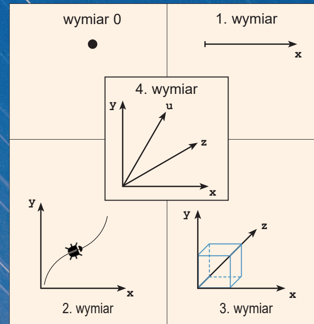
Rysunek 1: Układy współrzędnych w różnych wariantach (wszystkie osie tworzą między sobą kąt 90°)
