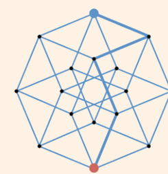
Rysunek 2: Projekt 4 – wymiarowej bryły
