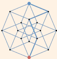
图2： 四维超立方体在二维空间上的投影。
