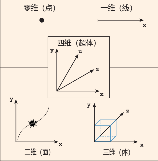
图1： 不同维度坐标系（所有轴互成90°）。
