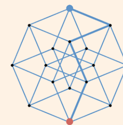
Bild 2: Projektion eines Würfels der 4. Dimension
