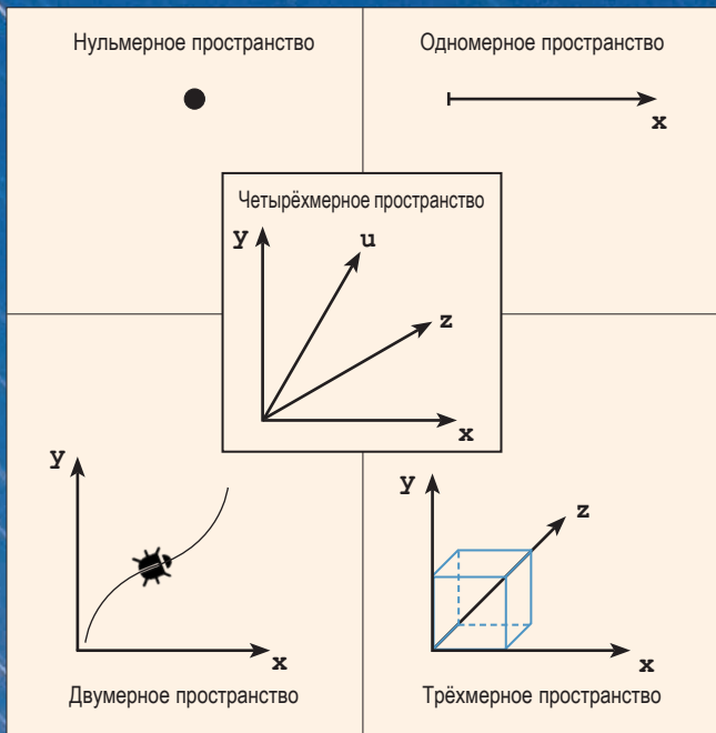
Рис. 1: Системы координат в различных измерениях (все оси координат располагаются под углом 90^\circ по отношению друг к другу)
