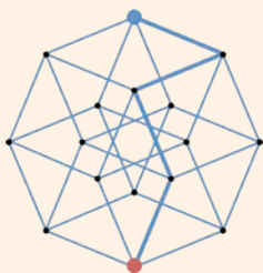
Рис. 2: Проекция 4-х мерного гиперкуба (куба четвёртого измерения) на плоскость
