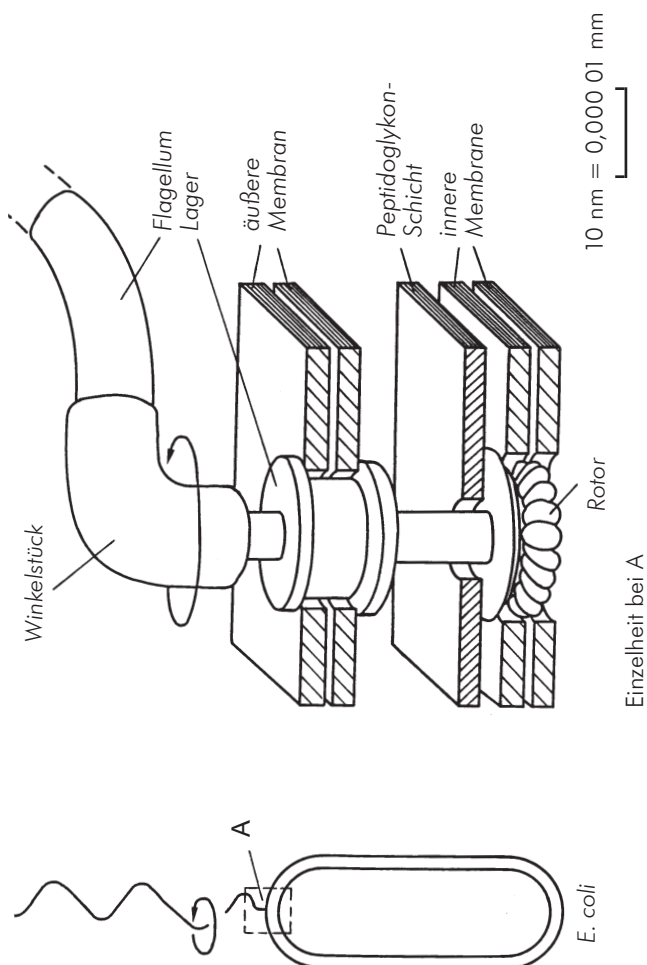
Bild 4: Escherichia coli – das bekannteste Bakterium. Die Schnittzeichnung verdeutlicht die Wirkungsweise des Motors, der das Fortbewegungsorgan (lat. flagellum = Geißel, Peitsche) antreibt.
